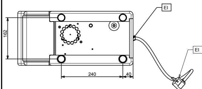
Boven aanzicht
